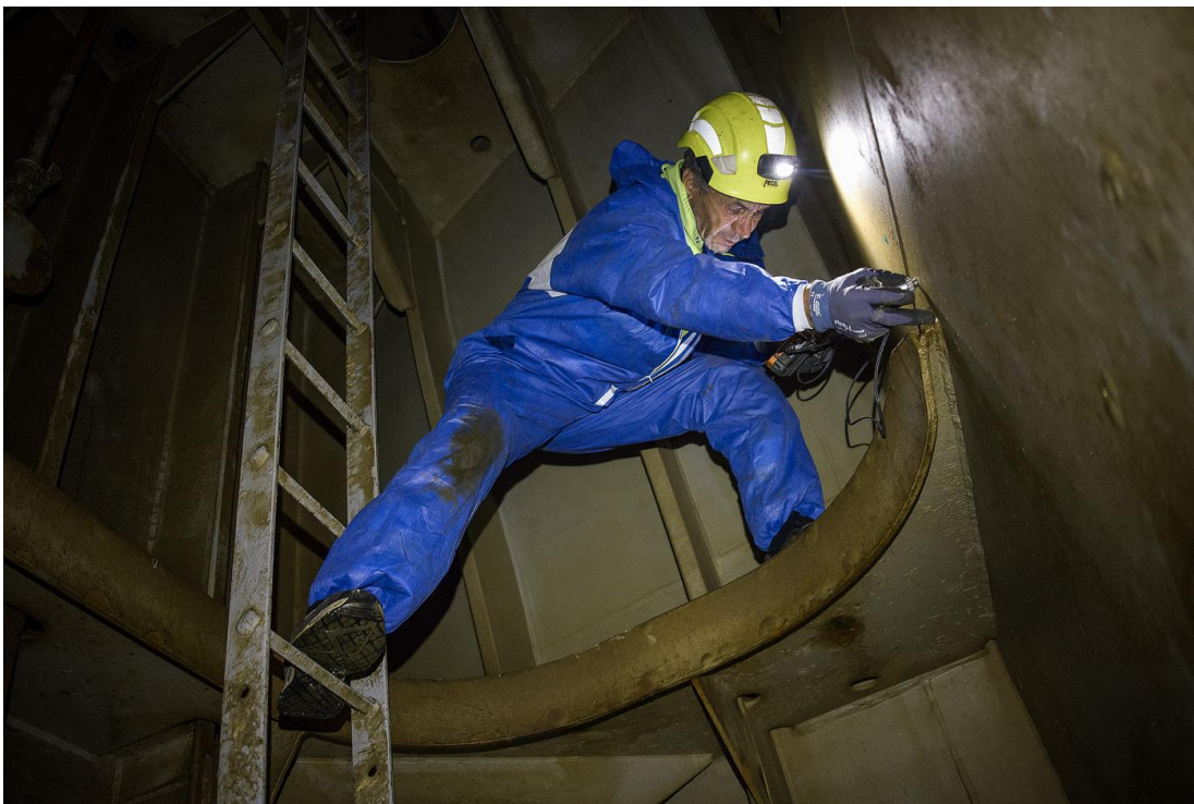
Dorel măsoară cu ultrasunete grosimea pereților și gradul de eroziune al unei nave. Portul din Odense, Danemarca
